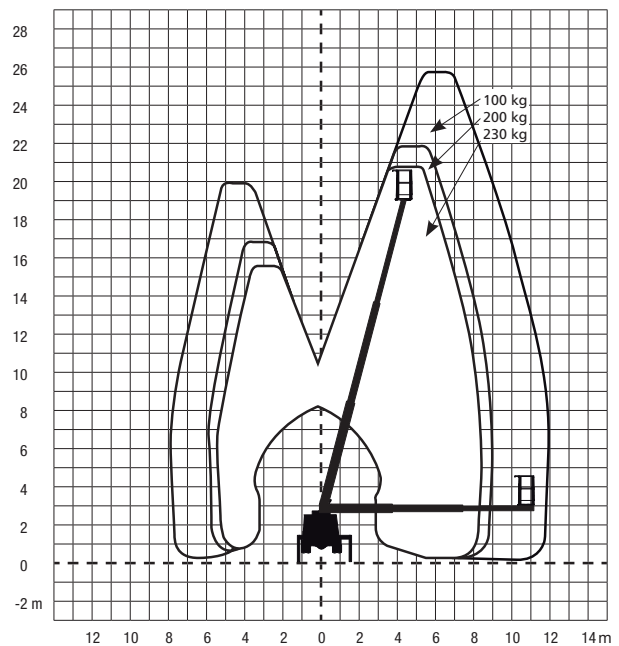
Bei einseitiger Abstützung nicht max. Arbeitshöhe
